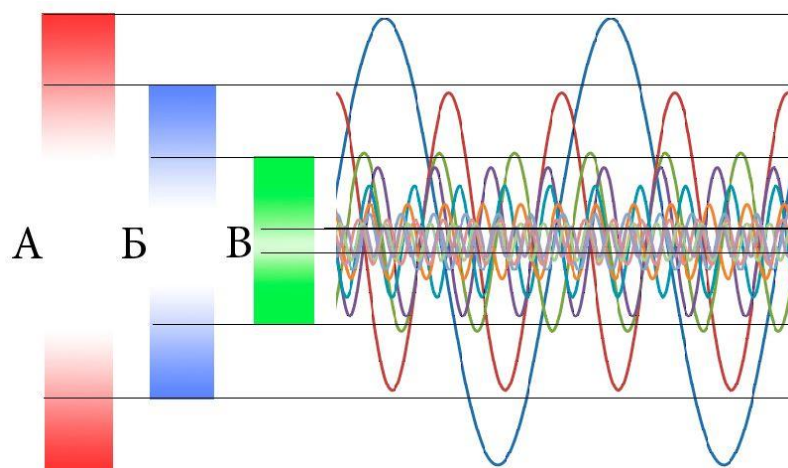
Рис. 84-1. Волновой пучок – то что мы увидим на практике
