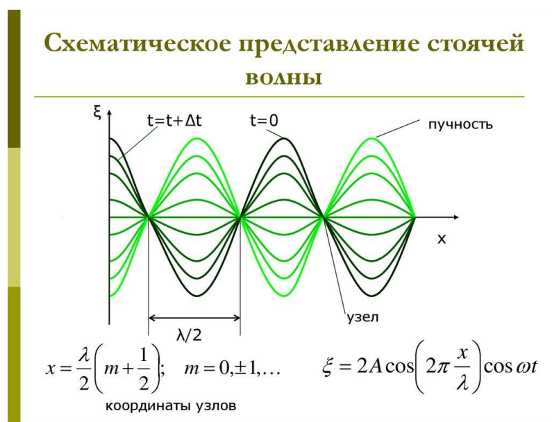
Рис. 84. Волновой пучок – теория. «Стоячая» электромагнитная волна.
