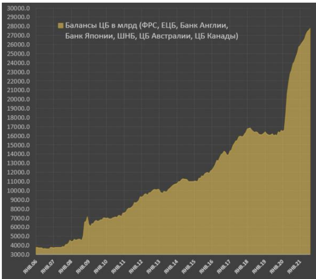
Рис.130. Динамика балансов ведущих мировых центробанков (без учета Народного банка Китая) 245
