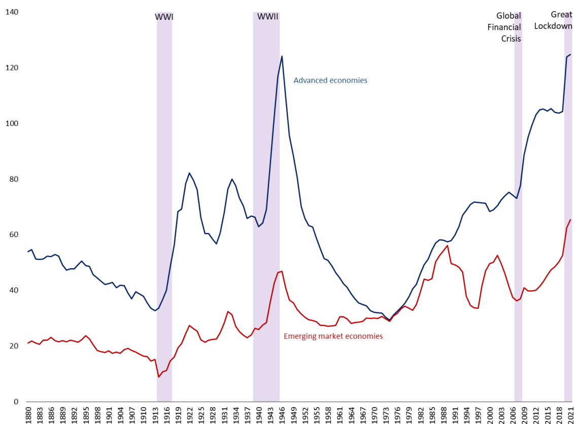
Рис. 131. Динамика показателя госдолг/ВВП по мировой экономике
